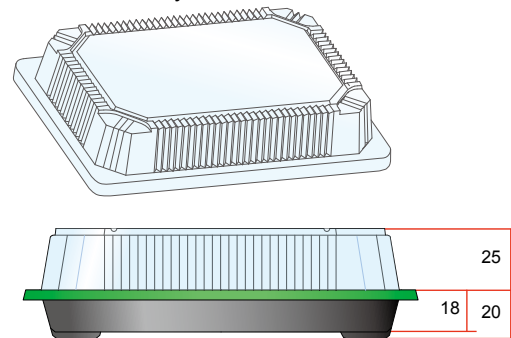
Economy Lid Lid-S
